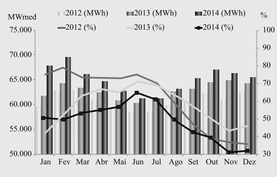
Gráf. 2 - Carga de demanda (barras) e média de energia armazenada (linhas) - SIN (Sistema Integrado Nacional)
