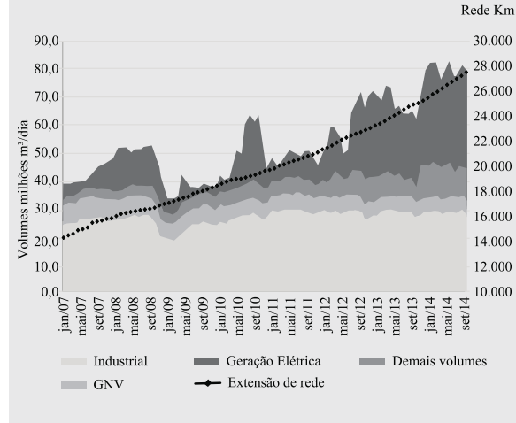
Gráf. 4 - Evolução do consumo e da extensão de redes de distribuição de gás natural - Brasil - 2007 a 2013
