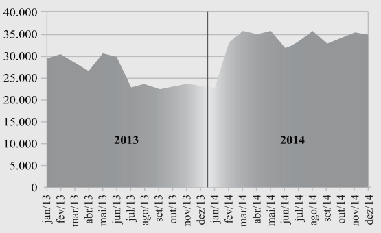
Gráf. 1 - Volume médio diário fornecido ao segmento termelétrico (m³)
